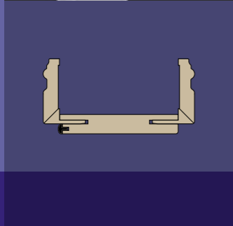
Profil B1 (65 mm)
