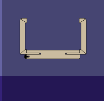
Rundkante (80 mm)
