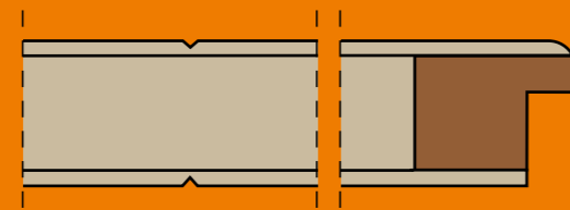
Querschnitt Tivoli
